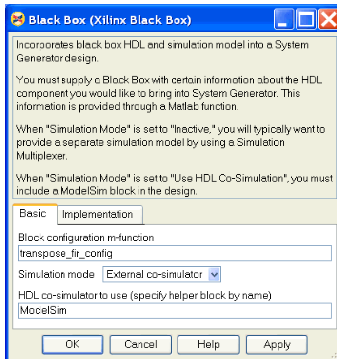
Figure 142: Black Box Parameters
