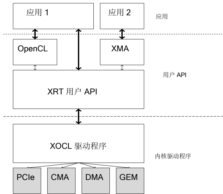
图 2.2: XRT 软件堆栈
