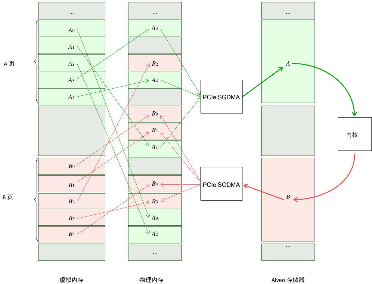
图 3.1: 虚拟内存与 Alveo 之间的数据传输
