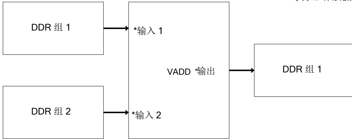
图 4.1：宽 VADD 内存连接
