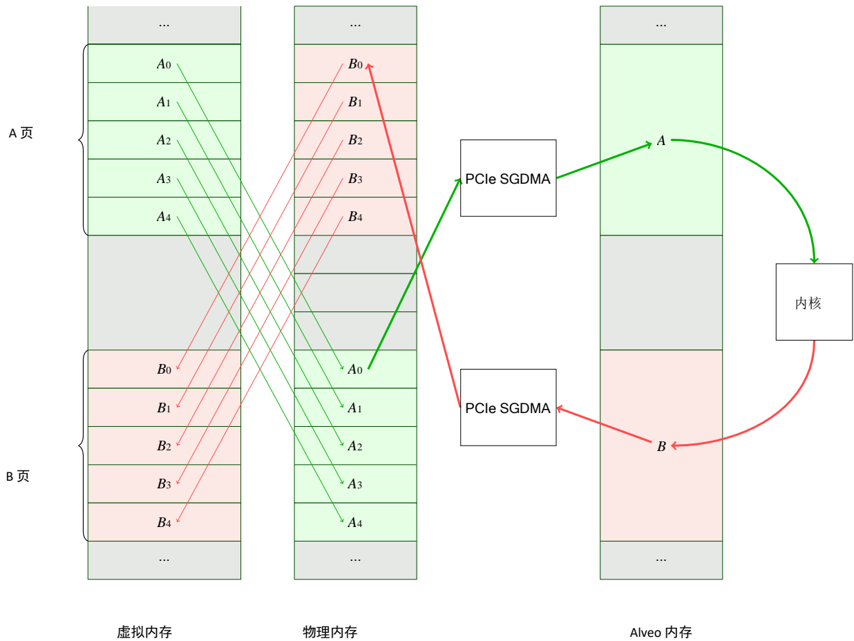
图 3.2: 虚拟内存与 Alveo 之间的数据传输
