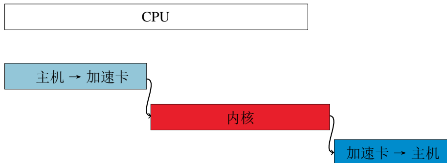
图 4.2：内核执行时间线
