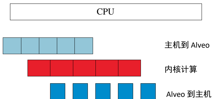
图 4.3：内核执行时间线（优化后）
