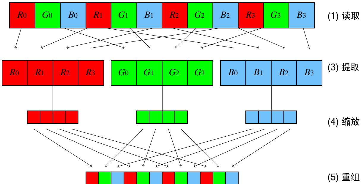
图 4.4: 缩放算法数据流
