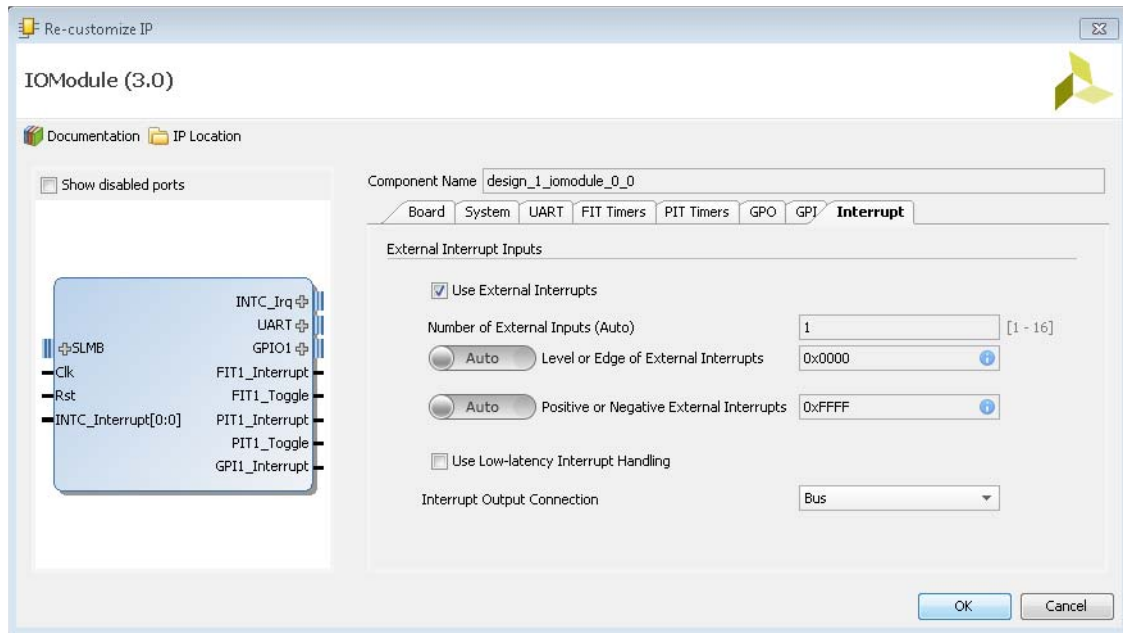
Figure 4-8: Interrupt Parameter Tab
