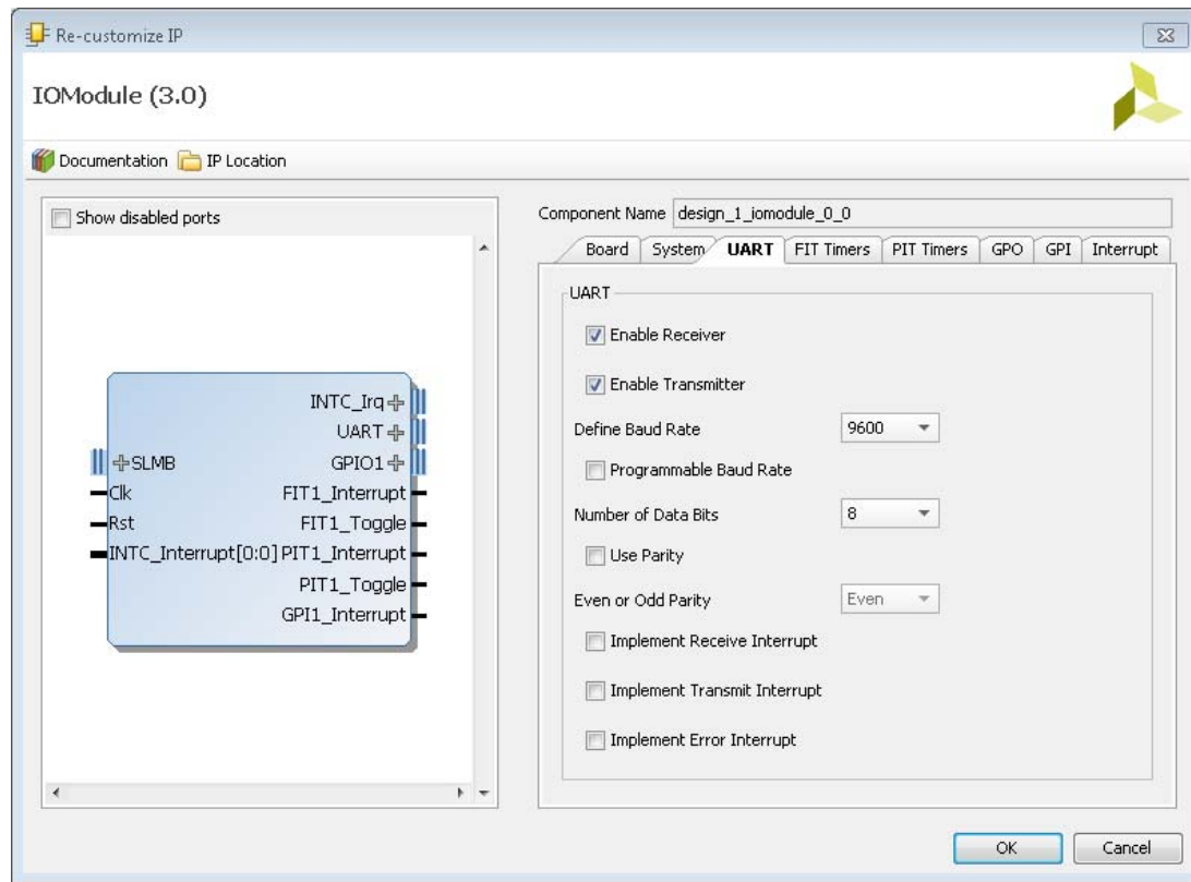
Figure 4-3: UART Parameter Tab
