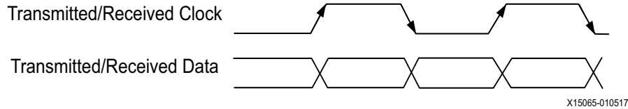
Figure 3-4: Edge DDR Strobe
